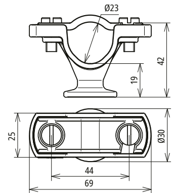
Maßbild LH ZS 23 H19 IGM8 GR PA
