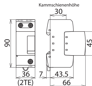
Maßbild DSE M 1 242
