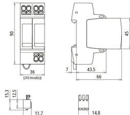
Maßbild DG MP TT 2P 385 FM
