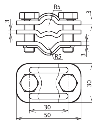
Maßbild UTK 7.10 7.10 S ZP STTZN
