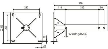
Maßbild SRS D50 300 300 H500 STTZN
