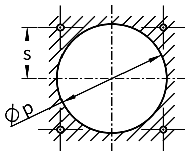
Montageausschnitt/ Mounting cutout
