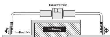
Prinzipschaltbild EXFS 100 KU
