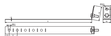
Maßbild RRS V 60.100 B10.5 CU
