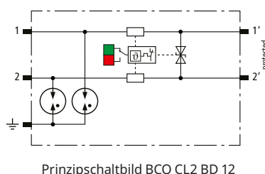
Prinzipschaltbild BCO CL2 BD 12
