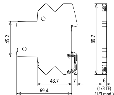
Maßbild BCO CL2 BD 12
