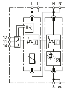
Prinzipschaltbild DG MP TT 2P ACI 275 FM
