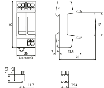
Maßbild DG MP TT 2P ACI 275 FM
