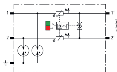
Prinzipschaltbild BCO ML2 BPD 24
