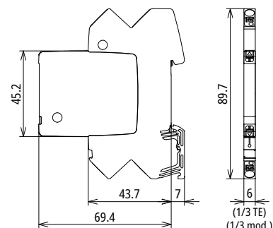
Maßbild BCO ML2 BPD 24
