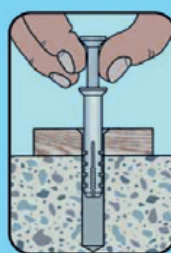
Dübel durch das Bauteil in Bohrloch stecken
