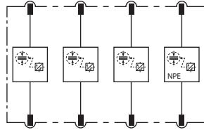
Prinzipialschaltbild DV MOD TT 255
