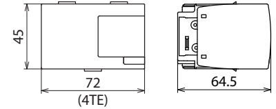
Maßbild DV MOD TT 255
