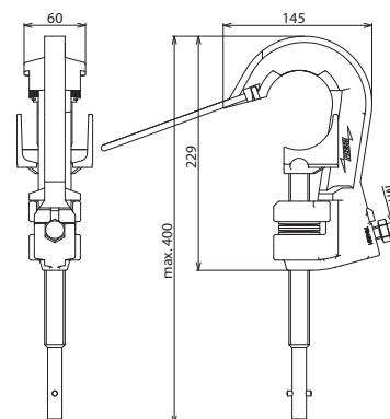
Maßbild PSK 10 65 SQL EH
