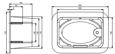
Maßbild UFTSK 300X220X120 GG
