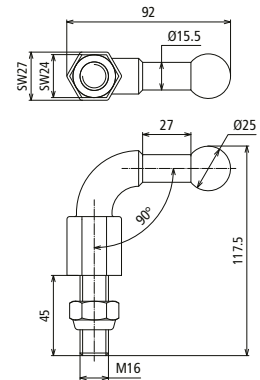
Maßbild KFP 25 W90 M16 45SSM
