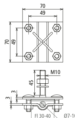
Maßbild AK 7.10 FL40 GBM10X45 STTZN
