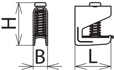
Maßbild SAK 11 SN MS
