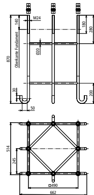
Maßbild AKO TBM FP565
