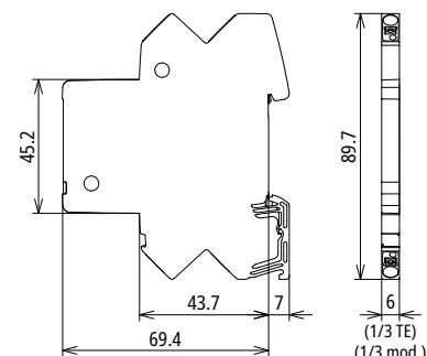
Maßbild BCO CL2 BE 12
