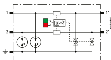
Prinzipschaltbild BCO CL2 BE 12
