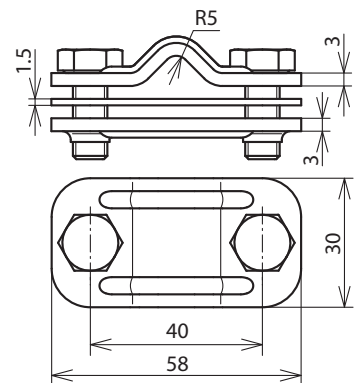
Maßbild ZMTK 8.10 FL30 CU STTZN
