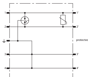
Prinzipschaltbild BXT M2 BD HC5A 24
