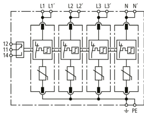
Prinzipschaltbild DG MD TNS 385 FM
