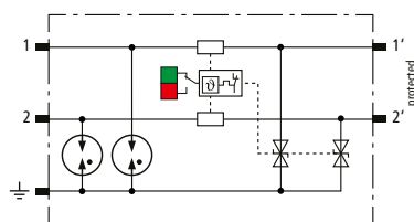
Prinzipschaltbild BCO MOD ML2 BE 24
