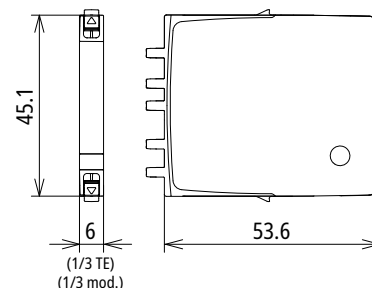
Maßbild BCO MOD ML2 BE 24
