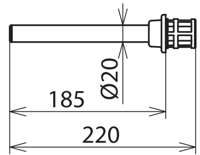
Maßbild L71 PS PHE 185
