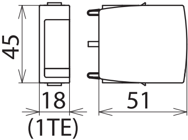
Maßbild DG MOD PV 500
