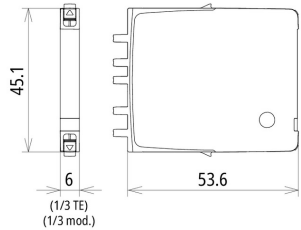
Maßbild BCO MOD ML2 BD 12
