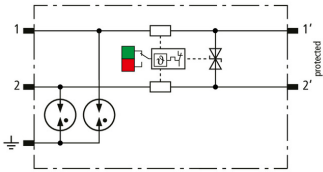
Prinzipialschaltbild BCO MOD ML2 BD 12
