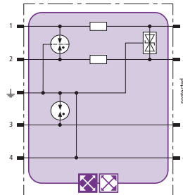
Prinzipschaltbild BXT ML2 BE HFS 5
