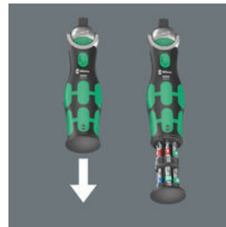
Im Griff der kompakten Zyklus Knarre ist ein unverlierbares, frei schwenkbares Bit-Magazin für 12 Bits (1/4", 25 mm Länge) integriert.
