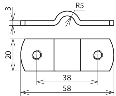
Maßbild ZSUEL 7.10 2XM6 LA38 AL
