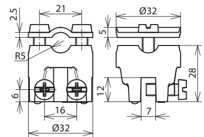
Maßbild FK ZS 7.10 KBF0.7 6 RG
