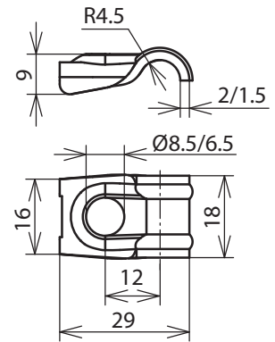
Maßbild UEL DQ 6.10 B6.5 V2A
