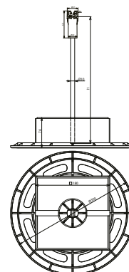
Maßbild DIDLH 8 H295 D300 BS
