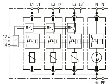
Prinzipschaltbild DG MD TNS ACI 275 FM
