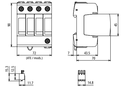
Maßbild DG MD TNS ACI 275 FM
