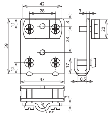
Maßbild FK ZS 7.10 KBF0.7 10 CU
