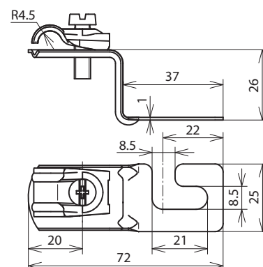
Maßbild DLH DQ 6.10 WPRO5 8 V2A
