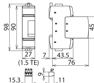
Maßbild DG SE CI 440 FM
