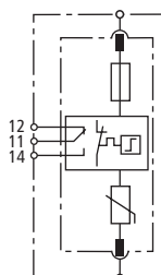
Prinzipialschaltbild DG SE CI 440 FM
