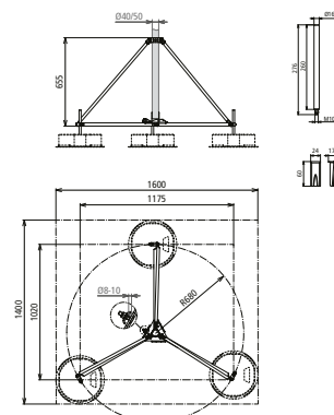
Maßbild DBS KB D50 RA680 V2A
