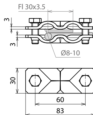
Maßbild SVPK 8.10 8.10 FL30 V4A
