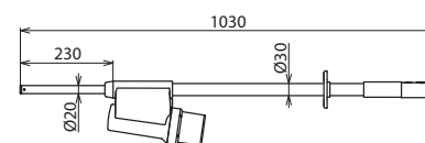
Maßbild PHE4 3 S
