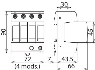
Maßbild DG MU 3PY 480 4W+G
