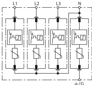
Prinzipschaltbild DG MU 3PY 480 4W+G
