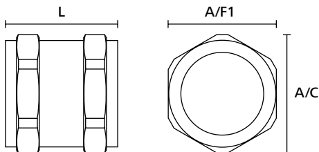
HelaGuard Anschlussverbinder
