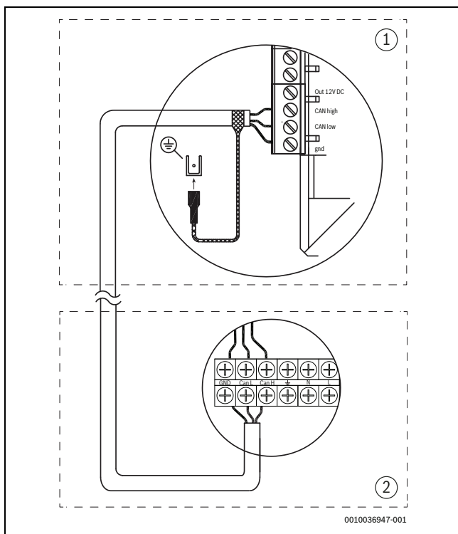
Bild 20 CAN-BUS-Verbindung
