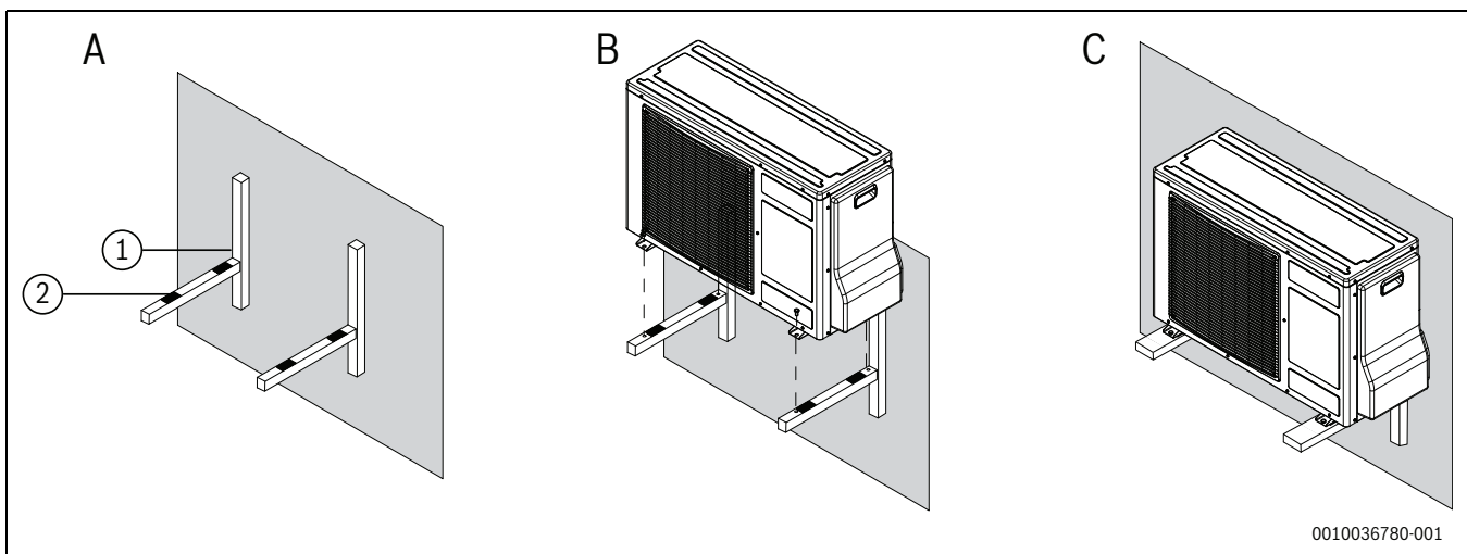
Bild 8 Wandhängende Außeneinheit
