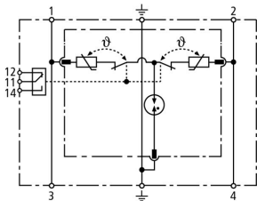
Prinzipialschaltbild DR M 2P 60 FM
