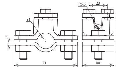
Maßbild ERS 42 AS4.10 TG STTZN
