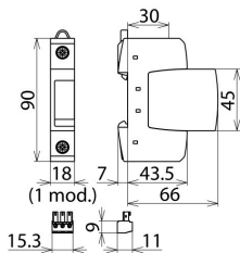
Maßbild DG SU 1P 240 R
