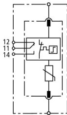
Prinzipschaltbild DG SU 1P 240 R
