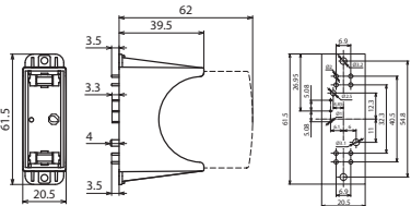
Maßbild DG PCB PV 500 FM
