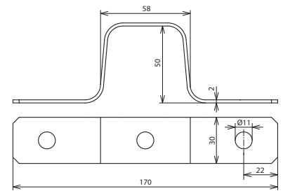
Maßbild DS 30X2 L170 3XB11 AL
