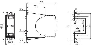
Maßbild DG PCB PV SCI 300
