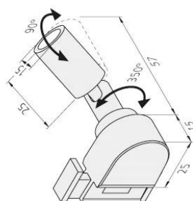
Glasbodenhalter
